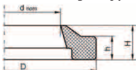
Pierścienie zgnajające
